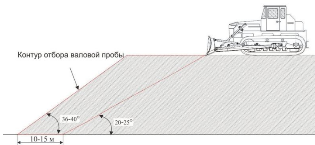
Рис. 0.15 Схема отбора валовых проб с помощью бульдозера
